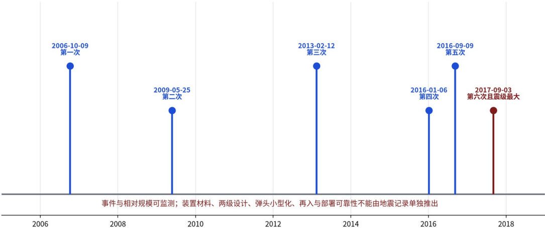
图4 CTBTO记录的朝鲜六次核试验相关事件（2006—2017）
